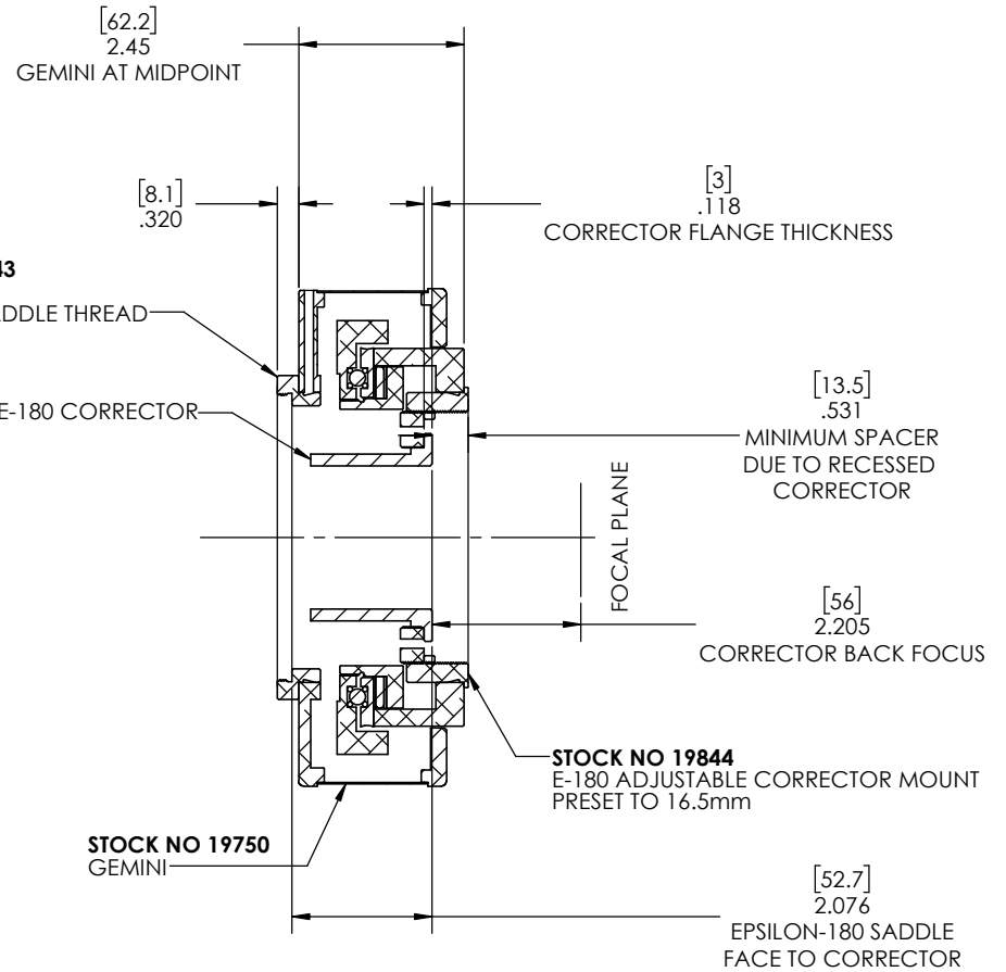
SECTION A-A
