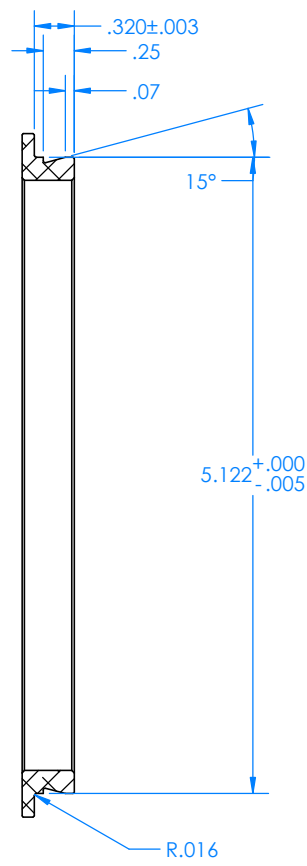
SECTION A-A
